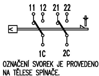
SCHEMA ZAPOJENÍ PŘI TEPLITĚ ČIDLA 20°C
